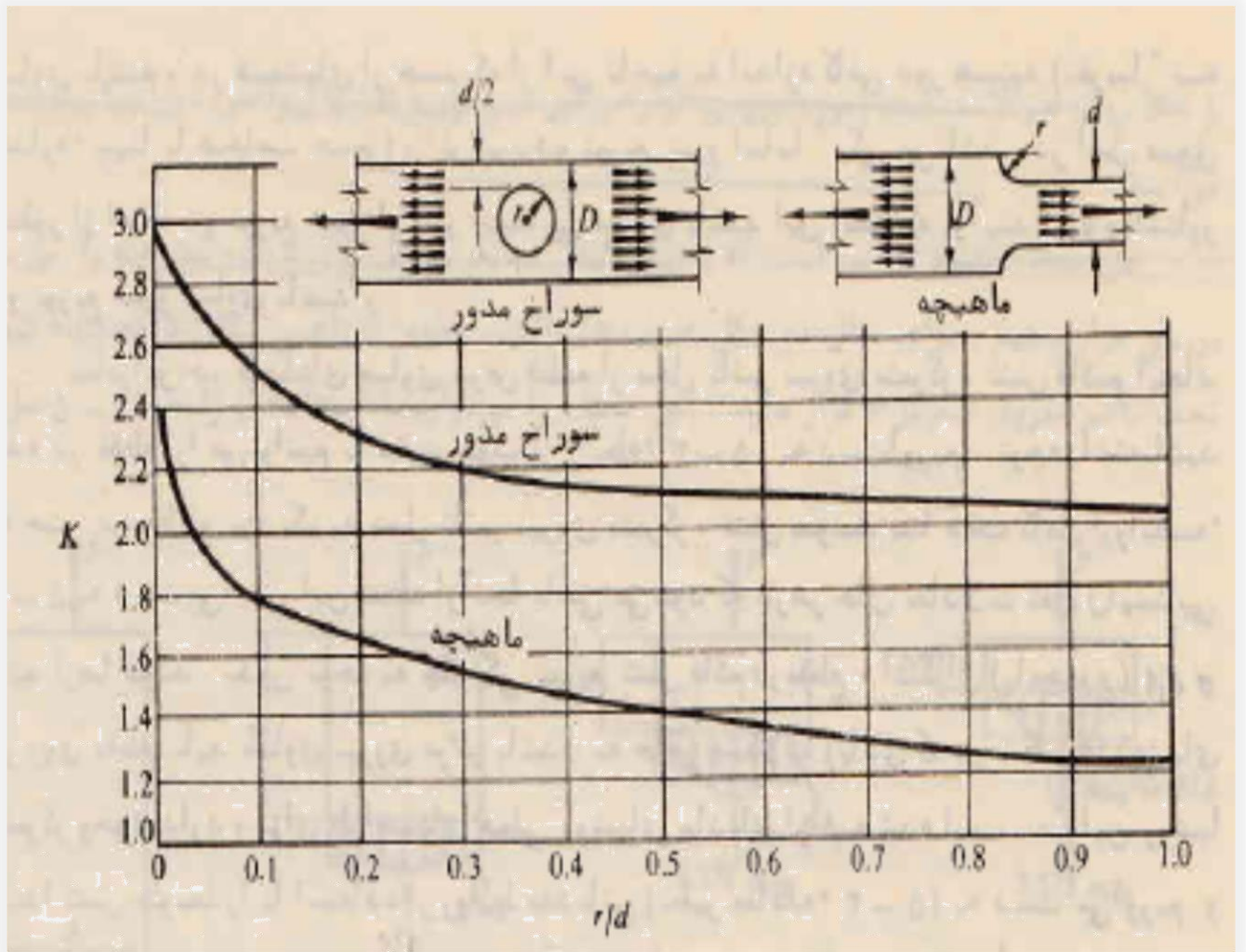
جدول محاسبه ضریب تمرکز تنش برای دو نمونه سوراخدار و ماهیچه
